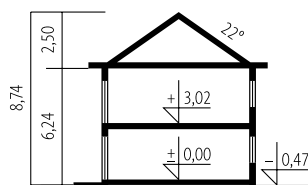
Schemat przekroju
