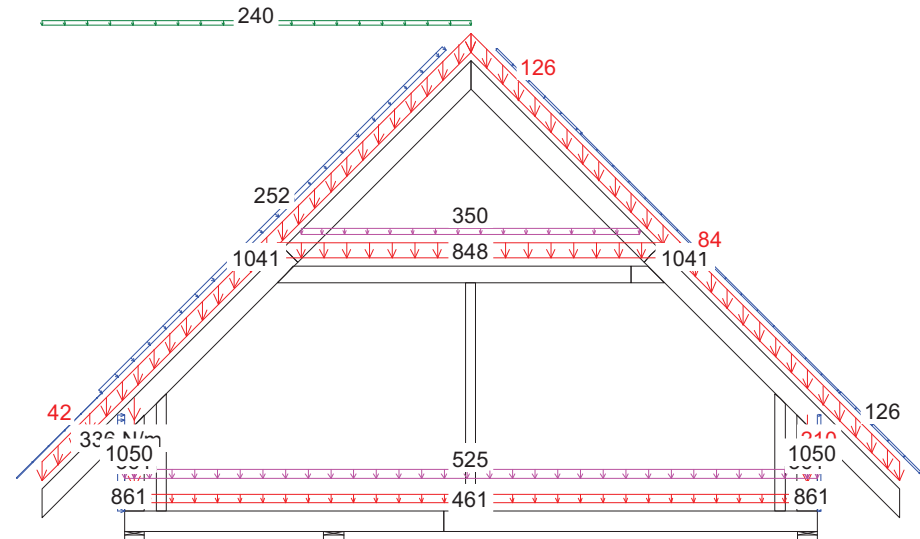
31 Kr Stale + 0.7*(OZ1 + OZ2 + OZ3) + 0.5*ŚniegL(0P) + WiatrL, Winst
