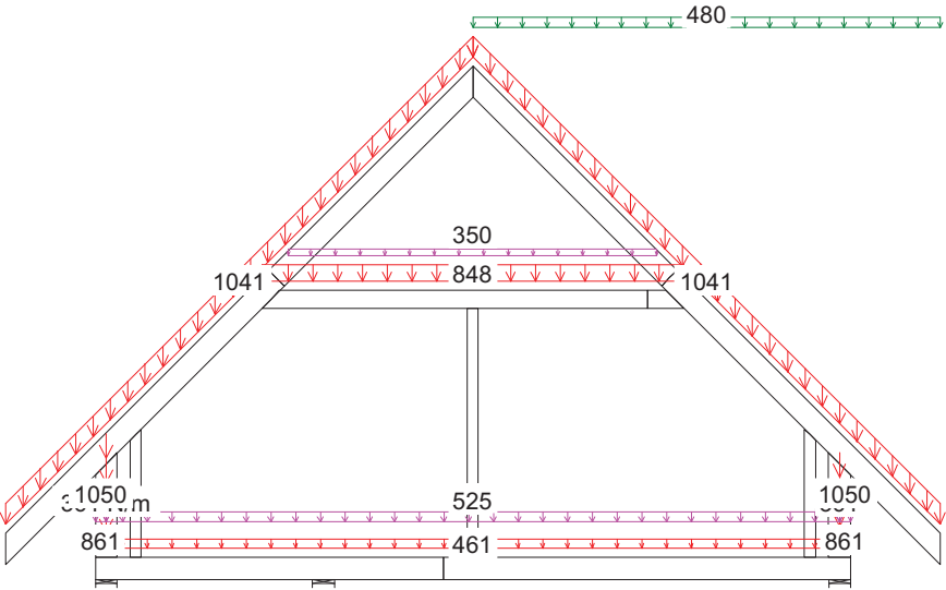
21 Śr Stałe + ŚniegP(0L) + 0.7*(OZ1 + OZ2 + OZ3), Winst
