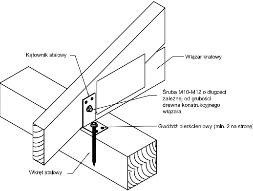
Schemat montażowy połączenia wiązara z murlatą
