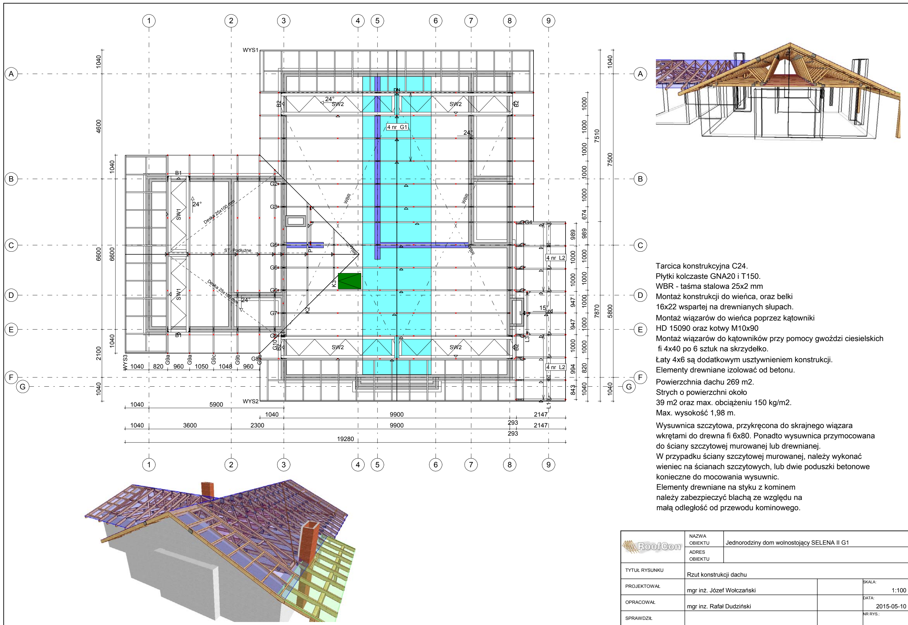
Prefabrykowana więźba dachowa - dom parterowy SELENA II G1
